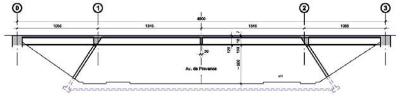
COUPE B-B 1:250
